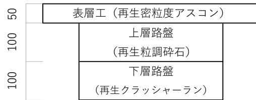
N3 (旧L交通) 一般的な町道
