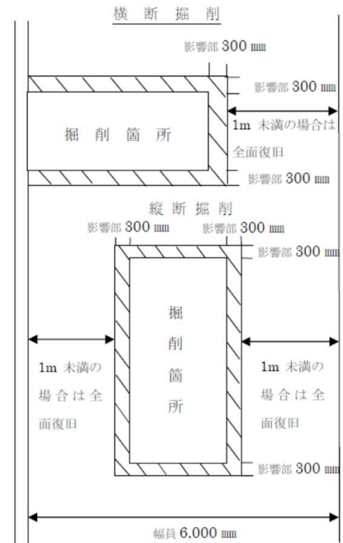
舗装道復旧断面図
